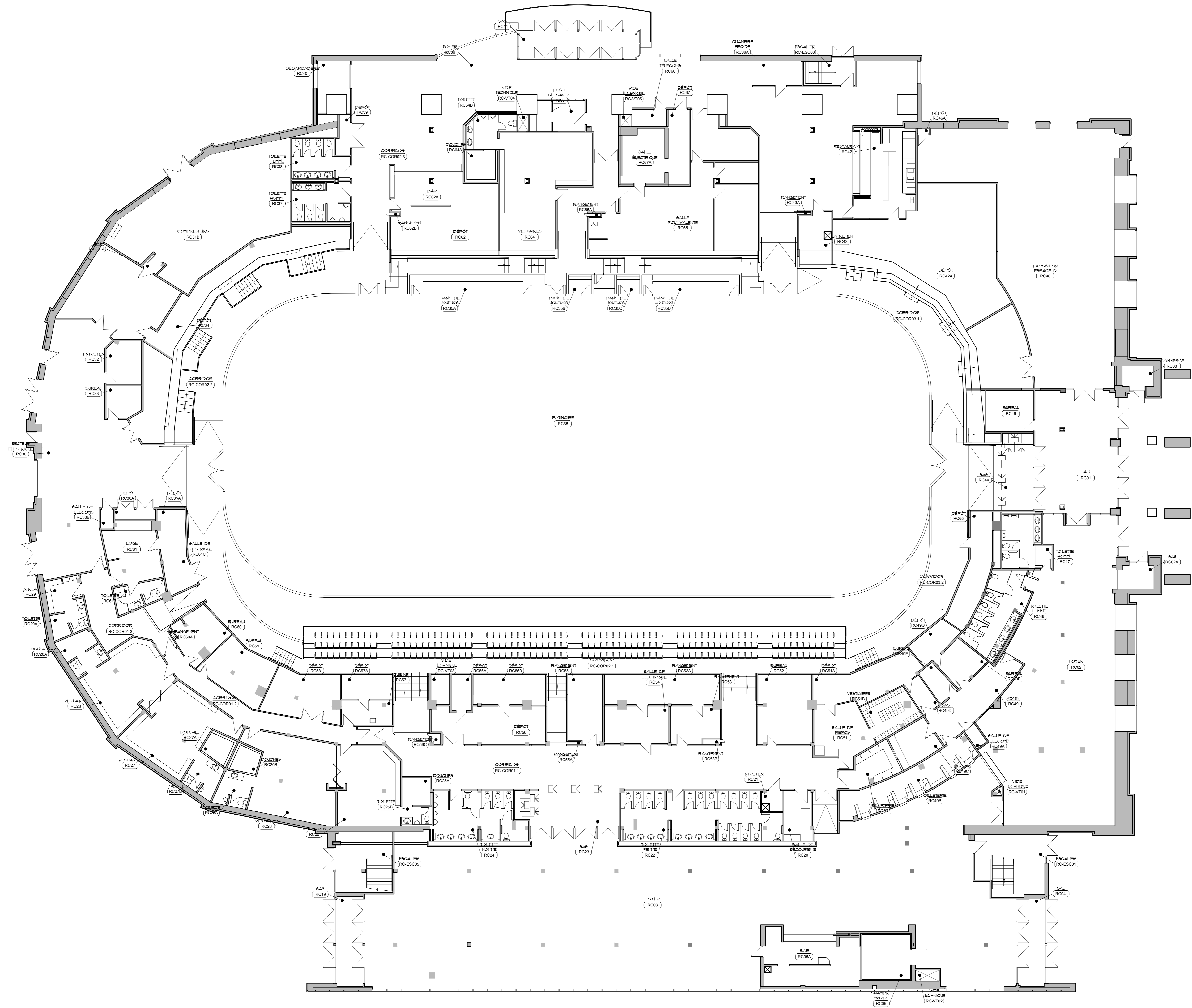
PLAN REZ-DE-CHAUSSÉE ÉCHELLE : 1:125
